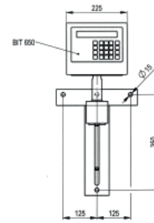
Frontansicht MHW
